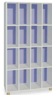
■ Mod.7422 casellario a giorno 16 vani dimensioni: cm.104x44x201h.
